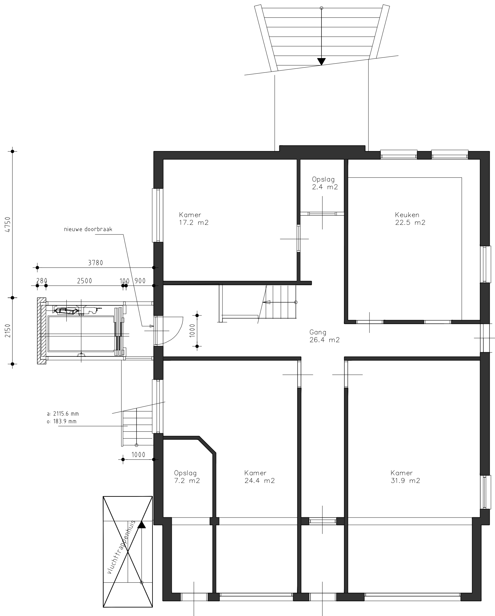
Plattegrond souterrain Nieuw
