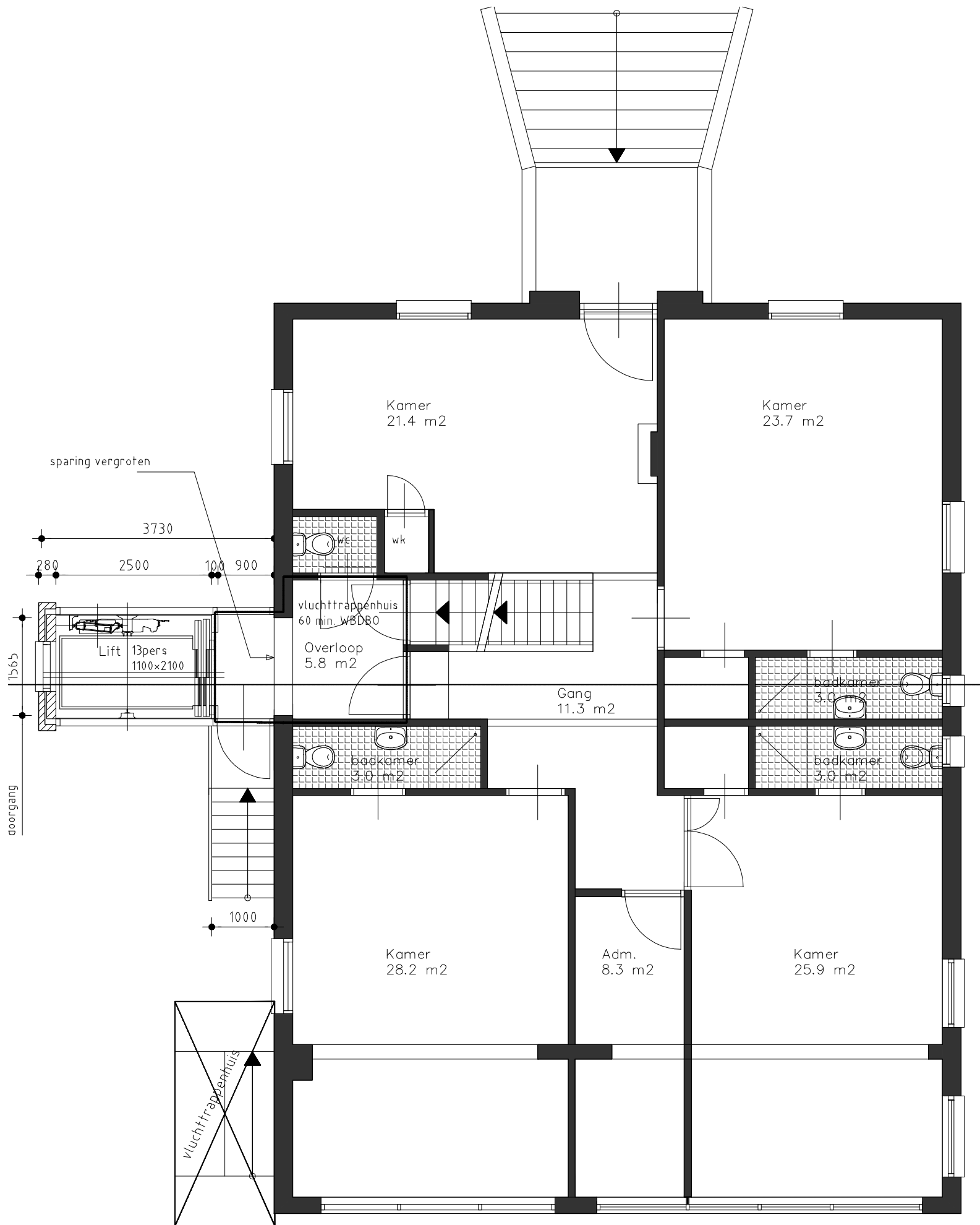
Plattegrond begane grond Nieuw
